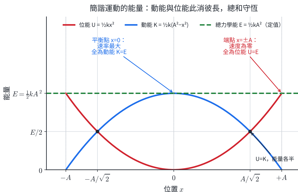
圖 5-4：簡諧運動的能量隨位置分佈。位能 U = \frac{1}{2}kx^2 為上凹拋物線（端點最高、平衡點為零），動能 K = \frac{1}{2}k(A^2 - x^2) 為下凹拋物線（與 U 相反），兩者在 x = \pm A/\sqrt{2} 處各佔一半；任意位置兩者相加皆為定值 E = \frac{1}{2}kA^2 （水平線），即總力學能守恆。
