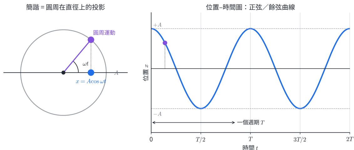
圖 5-5：左——半徑 A 、角速度 \omega 的等速圓周，其在 x 軸上的投影為 x = A \cos \omega t ；右——投影隨時間描出餘弦曲線，一個來回對應圓周轉一圈，週期同為 T = 2\pi/\omega 。
