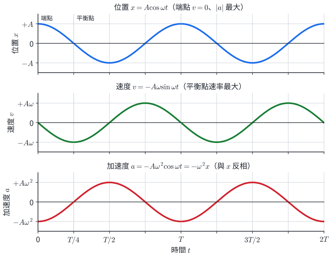
圖 5-3：簡諧的位置、速度、加速度對時間。 x 與 a 反相（一個到頂、另一個到谷，因 a = -\omega^2 x ）； v 比 x 提前 T/4 。端點（ x = \pm A ）時 v = 0 、 |a| 最大；平衡點（ x = 0 ）時 |v| 最大、 a = 0 ——「速度最大」與「加速度最大」發生在不同位置。
