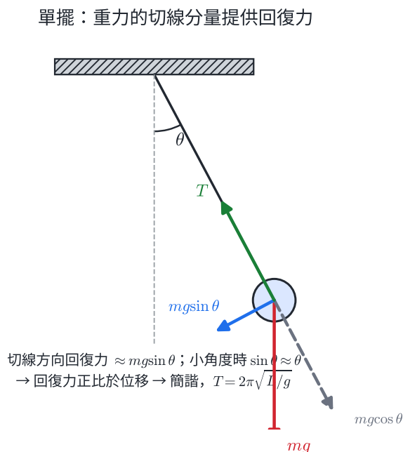
圖 5-6：單擺受力分解。重力沿擺線的分量 mg \cos \theta 與張力相關，沿切線的分量 mg \sin \theta 指向平衡位置，即為回復力；小角度時 \sin \theta \approx \theta ，回復力近似正比於位移，故近似為簡諧。
